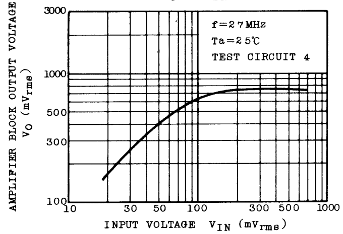
V_o - V_{IN}
