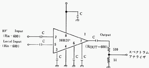
図 1. 測定回路
