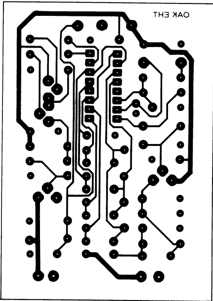
Fig. 8-c: Print van de ingangsversterker voor 10/50 MHz (A' en B).
