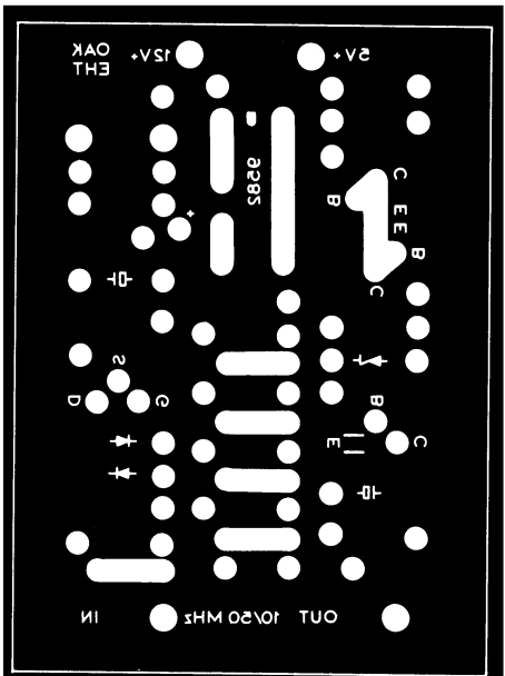
Fig. 8-p: Componentenrijde print ingangsverster- ker voor 10/50 MHz (A' en B).
