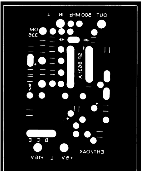
Fig. 7-p: Componentenrijde print voor de 500 MHz ingangsversterker-bescaler (A2)
