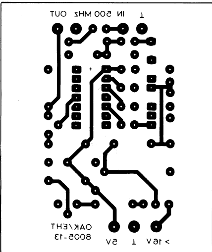
Fig. 7-c: Print voor de 500 MHz ingangsversterker- bescaler (A2)
