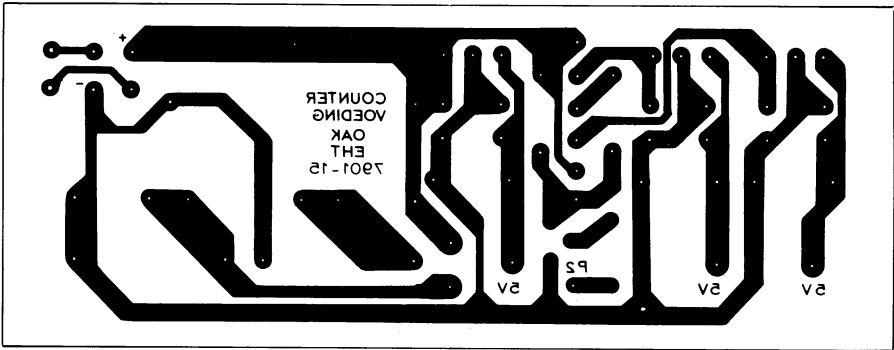
Fig. 8-d. Print van de voeding.
