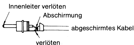
Abb. 3-4 Anbringung der RCA-Stecker
