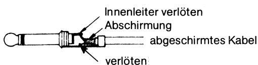
Abb. 3-3 Anbringung des Klinkensteckers
