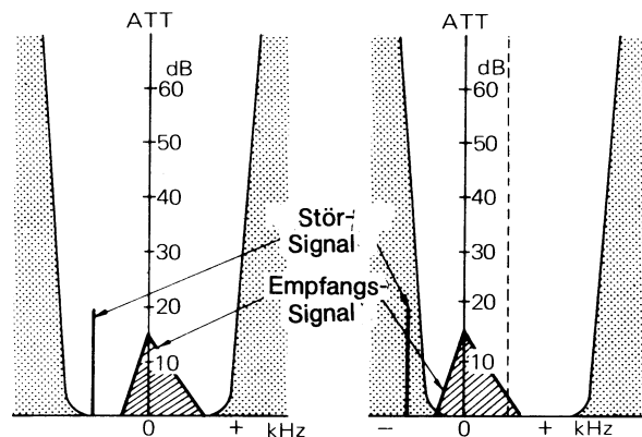
PBT-Regler in Mittelstellung
