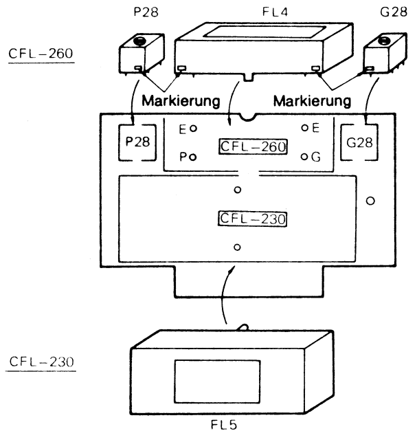
Montage der zusätzlichen Filter
