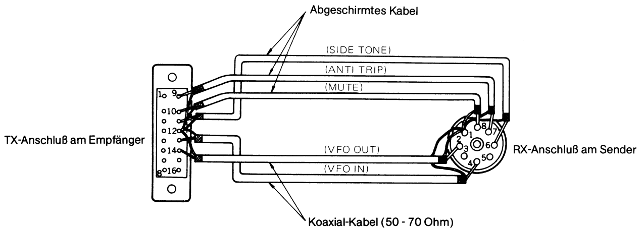
Abb. 5-5 Verbindungskabel für Sender und Empfänger (HF)
