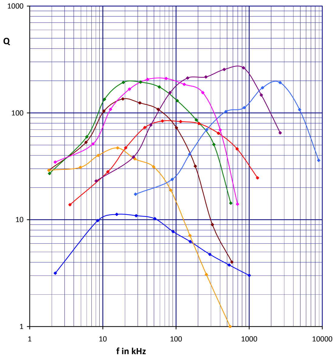
12 - 15 mm toroids - Q - N=25 3H1 , 3E25 , 3F3 , FT50-43 , FT50-77 , 4A11 , 4C65 , T50-2
