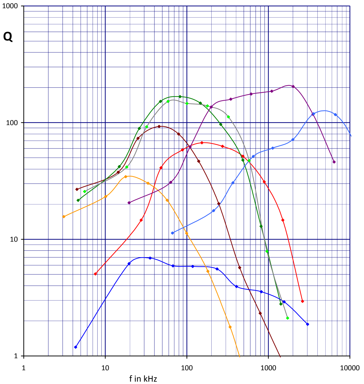
12 - 15 mm toroids - Q - N=10 3H1 , 3E25 , FT50-43 , FT50-77 , 3F3 , 4A11 , 4C65 , T50-2
