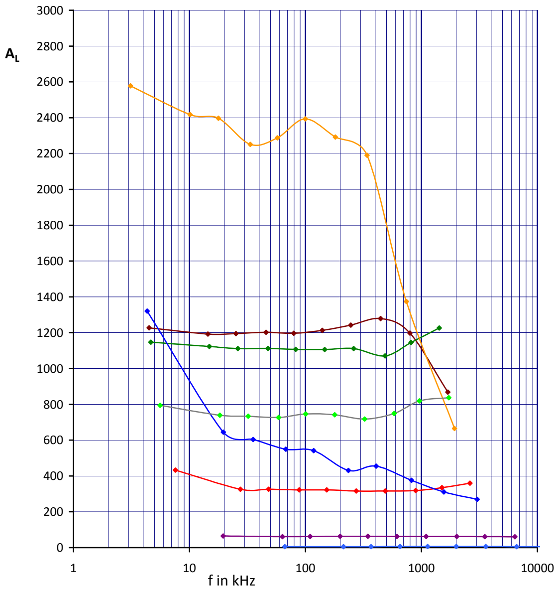
12 - 15 mm toroids - AL value - N=10 3H1 , 3E25 , FT50-43 , FT50-77 , 3F3 , 4A11 , 4C65 , T50-2
