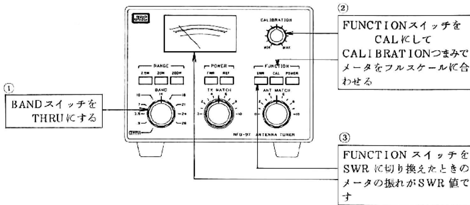
図 3.2 SWR測定の設定
