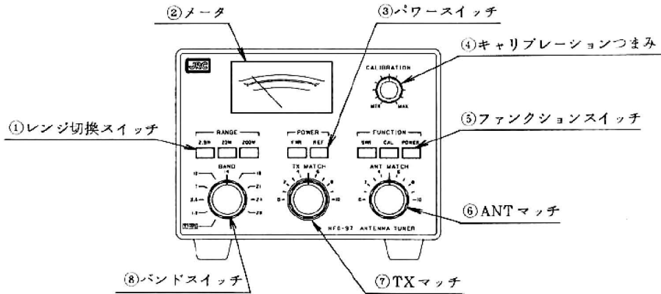
図 2.1 前面パネル
